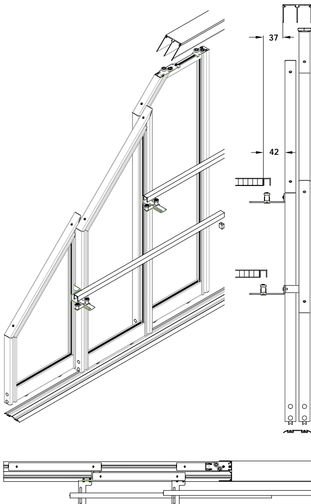
Länge = Türflügelbreite – 68 mm
