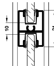
Länge = Türflügelbreite – 68 mm
